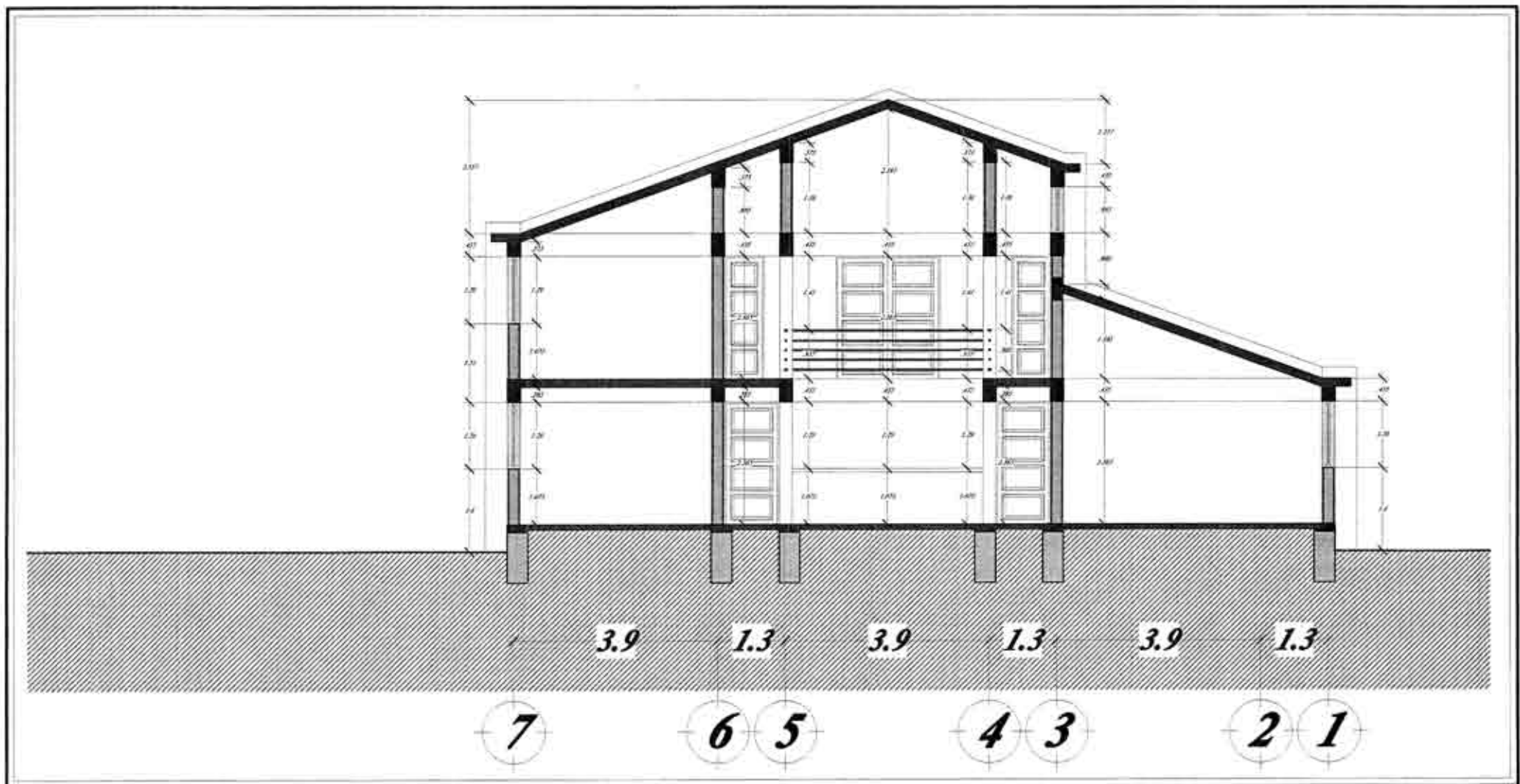
COUPE A-A
