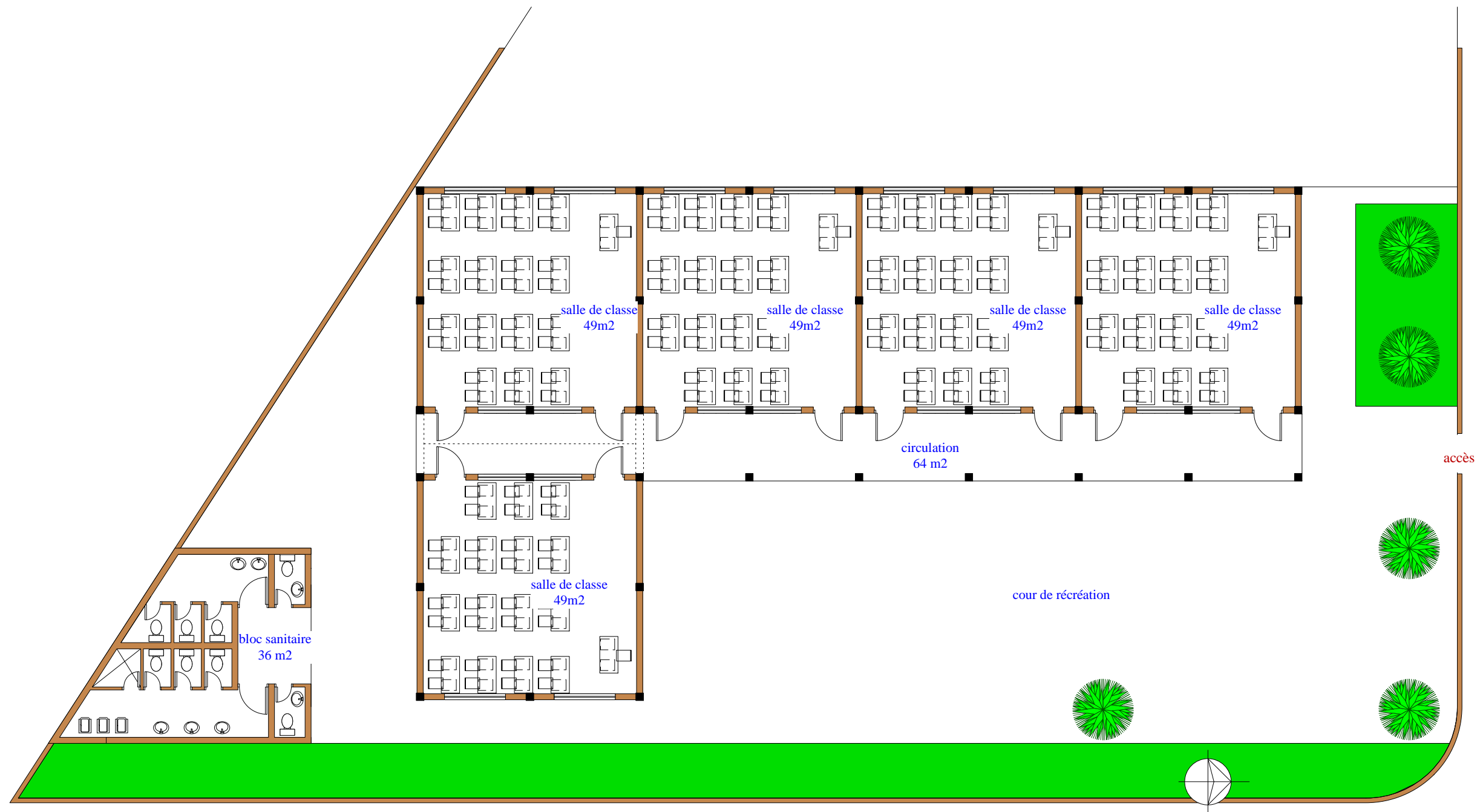
REZ-DE-CHAUSSÉE: PLAN D'ENSEMBLE ech.: 1/150
